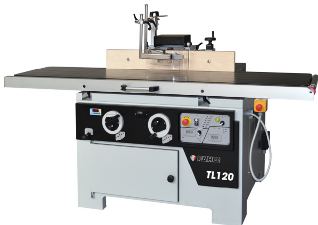
TL 120 versione con piani prolungati e albero inclinabile TL 120 version with long tables and tilting spindle
