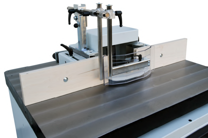
Cuffia toupie Movimentazione tramite volantini e spostamenti Visualizzati Spindle hood Linear movement by handwheels and displayed movements
